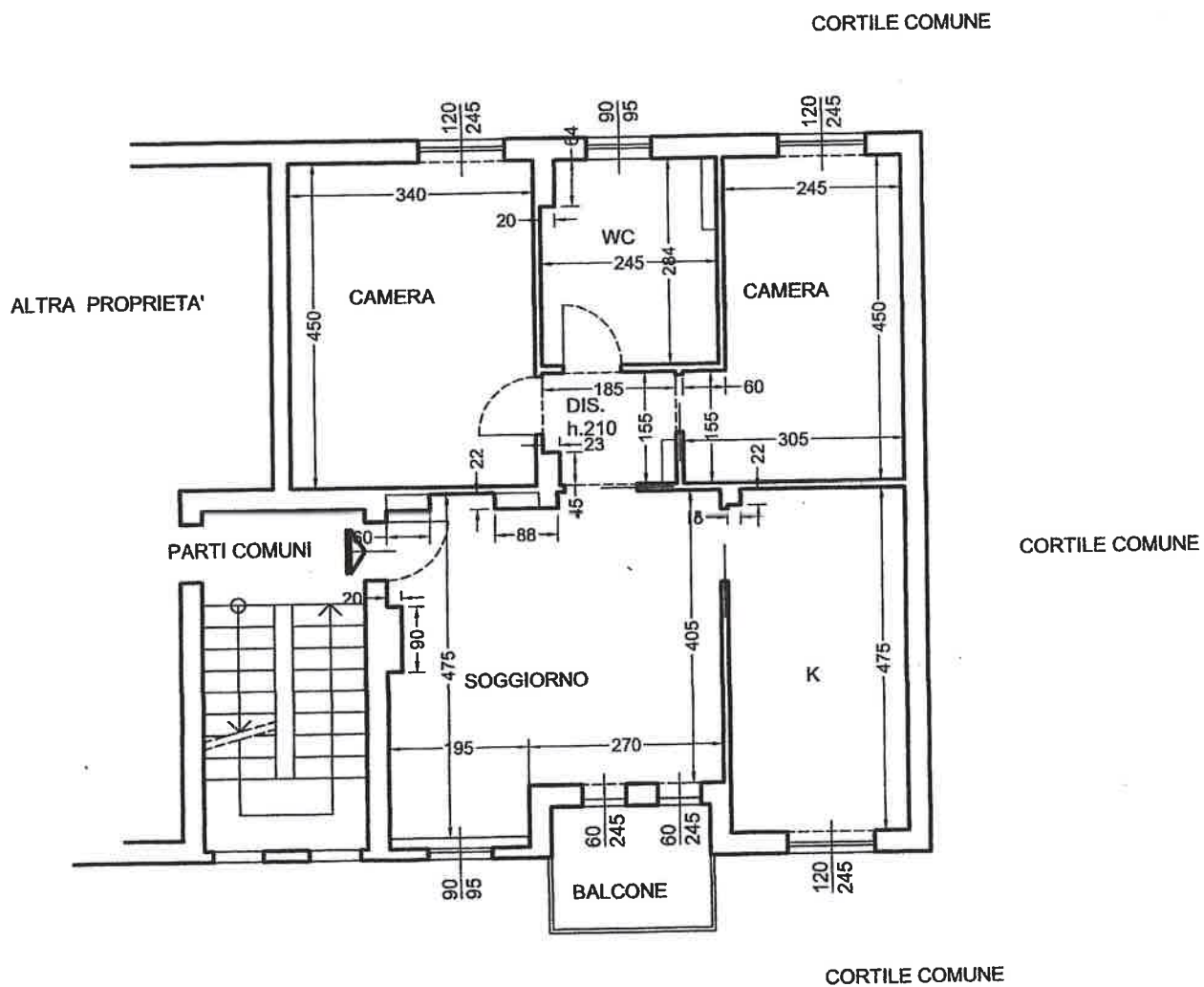
PIANTA PIANO SECONDO h.290
